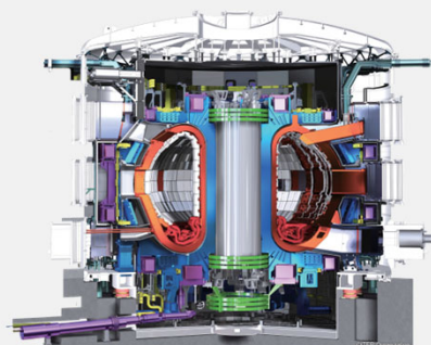
ITER外観図
